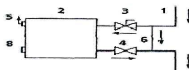
б - однотрубная система, подключение с перемычкой
