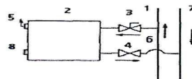
г - двухтрубная система, рекомендуемое подключение
